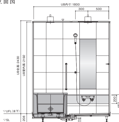
立面図
