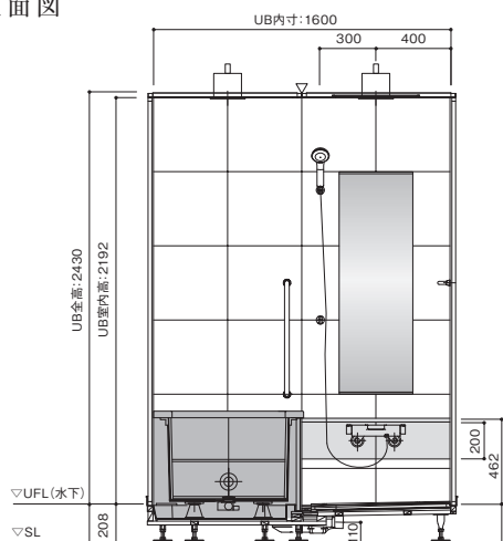
立面図
