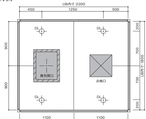
天井伏図
