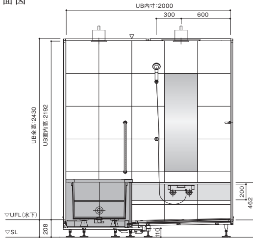
立面図
