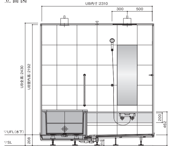
立面図
