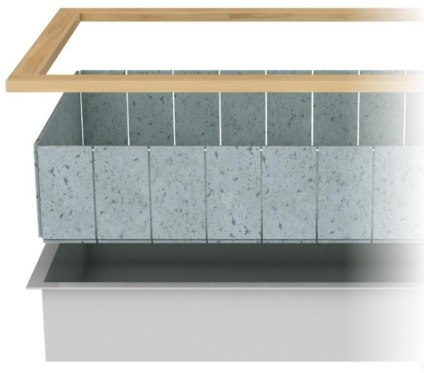
石貼り浴槽の構造イメージ
