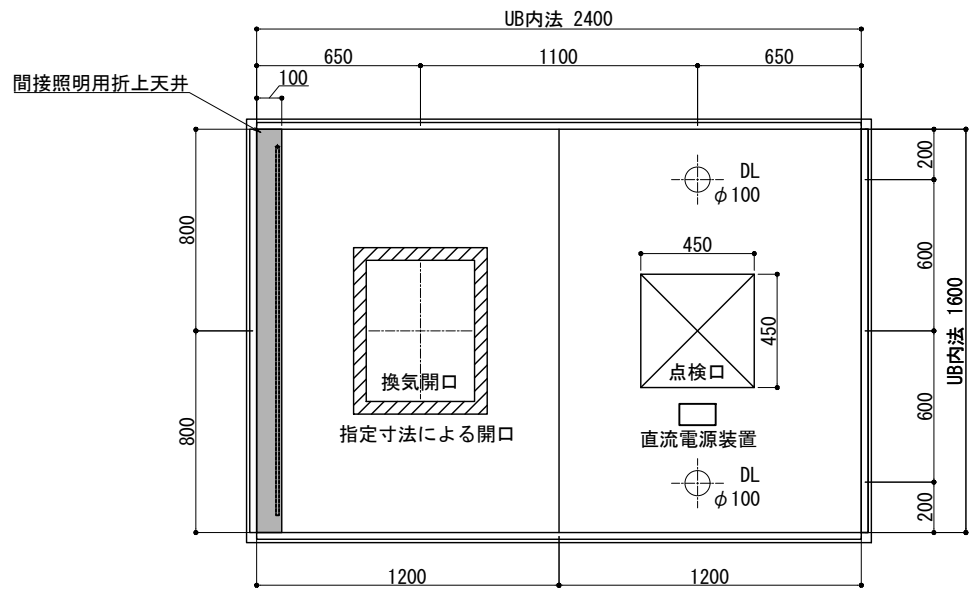
天井伏図
