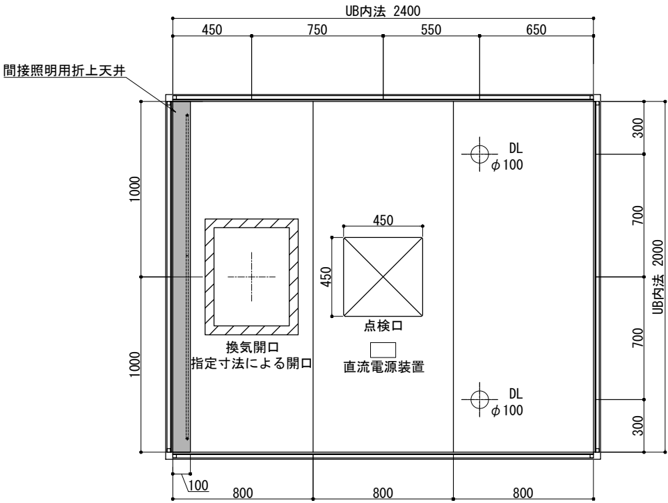
天井伏図
