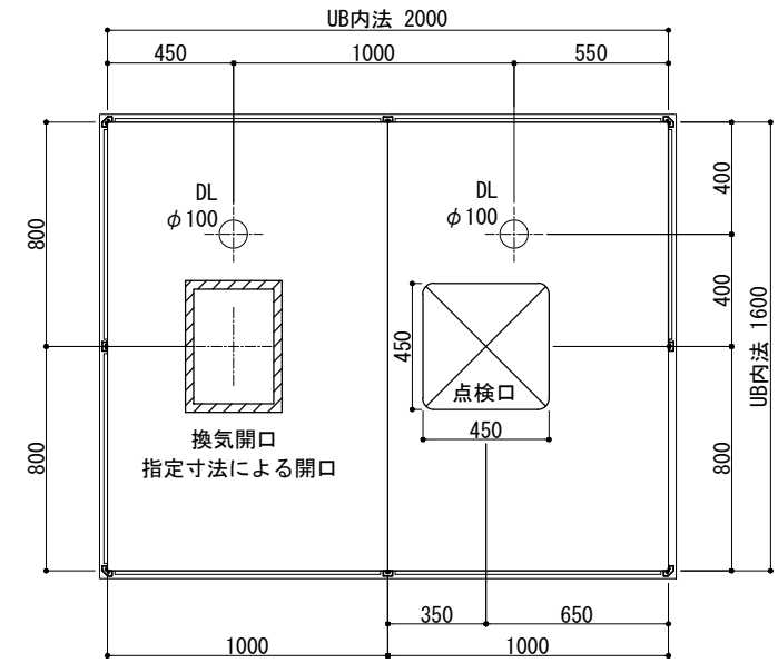
天井伏図
