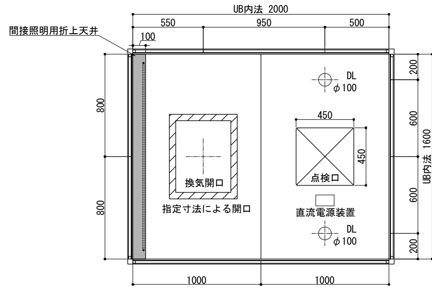
天井伏図
