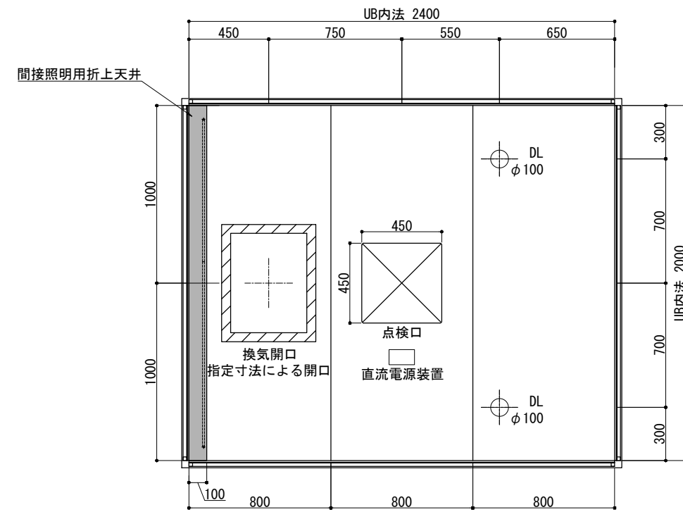
天井伏図
